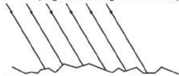
ଚିତ୍ର 16.6 ଅସମତଳ ପୃଷ୍ଠରେ ସମାନ୍ତରାଳ ରଶ୍ମିଗୁଡ଼ିକ ଆପତନ
