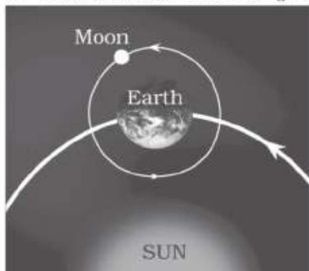
ଚିତ୍ର 17.4 ପୃଥିବୀର ଚନ୍ଦ୍ର ସହିତ ପୃଥିବୀ ଚାରିପଟେ ପରିକ୍ରମଣ
