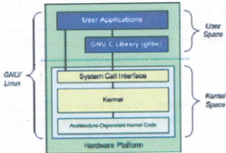
Fig. 1.6 Linux Kernel
