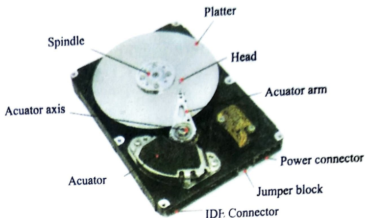
Fig. Hard Disk
