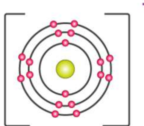
Chlorine ion Cl - - 2,8,8
