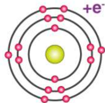
Chlorine atom Cl - 2,8,7
