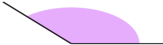
Obtuse Angle
