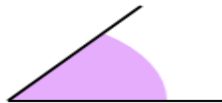
Acute Angle
