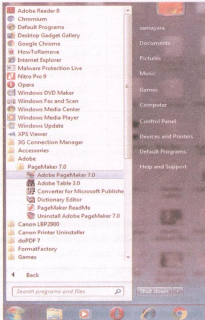
PageMaker Window
